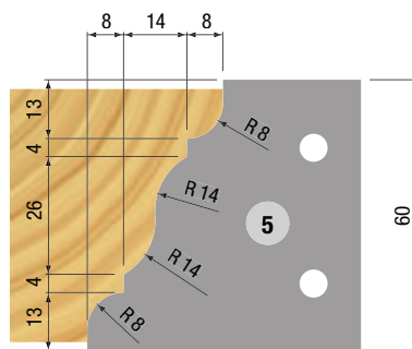
Profil 5 Cornice / Profile / Kranzprofil
