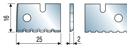
② Coltello / Knife / Messer
