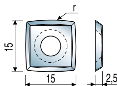
Coltello / Knife / Messer
