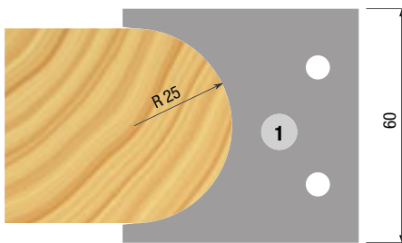
Profil 1 Mezzotondo / Half-round / Halbstab R 25
