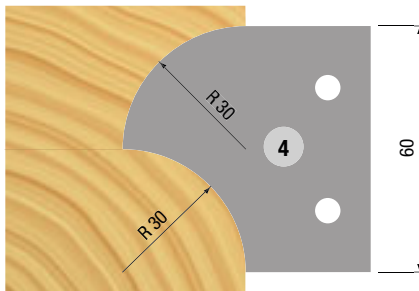
Profil 4 Doppio raggio / Dual-radius / Doppelradius R 30
