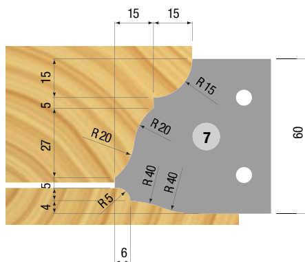
Profil 7 Profilo cornice/piattabanda Profile/panel rising Kranz/Abplatt geschweift
