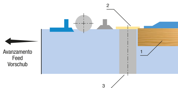
Vista dall'alto / Top view / Draufsicht von oben
