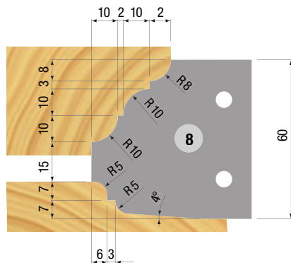
Profil 8 Profilo cornice/piattabanda Profile/panel rising Kranz/Abplatt gerade
