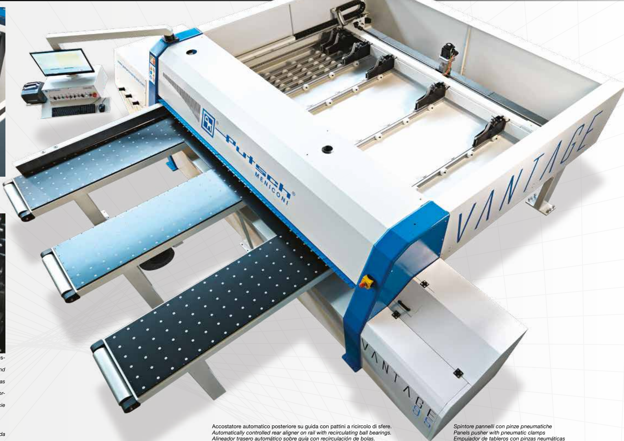
Motorizzazione spintore con Brushless e riduttore a ingranaggi (opt.) Brushless motor for pusher with reduction gear (opt.) Motor Brushless del empujador con reductor de engranaje (opt.) Brushless-Schiebomotor mit Untersetzungsgetriebe (auf Wunsch) Moteur Brushless du pousseur avec réducteur à engrenages (opt.)
