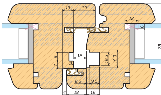
Sezione orizzontale - Chiusura centrale 78 Horizontal section - Central closure 78
