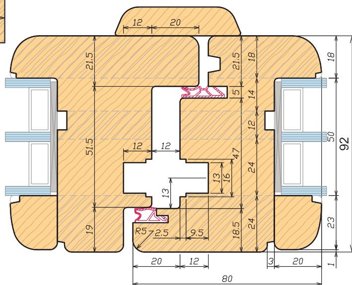
Sezione orizzontale - Chiusura centrale Horizontal section - Central closure
