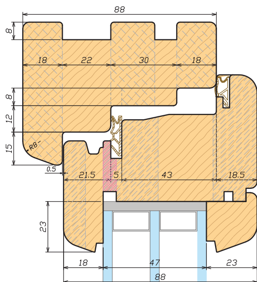
Sezione verticale 88 Vertical section 88
