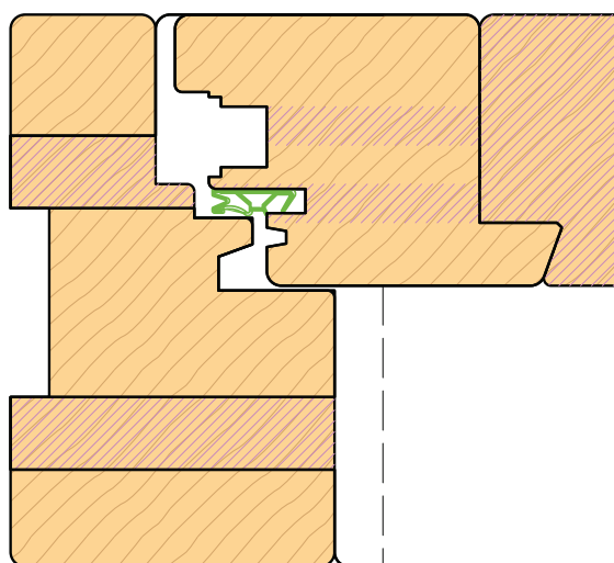
Sezione orizzontale Horizontal section
