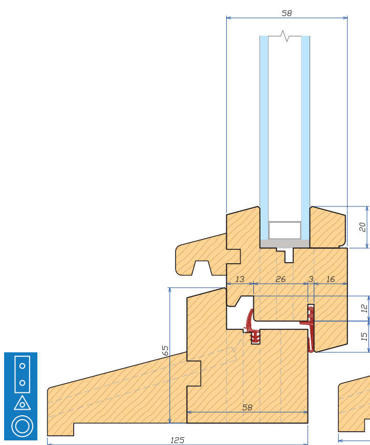
Sezione verticale 58 Vertical section 58
