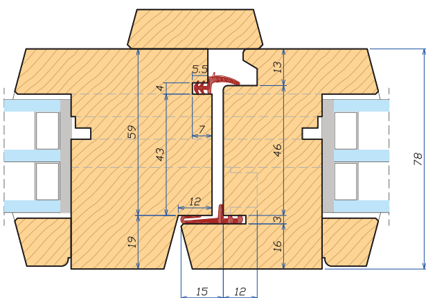
Sezione orizzontale - Chiusura centrale 78 Horizontal section - Central closure 78
