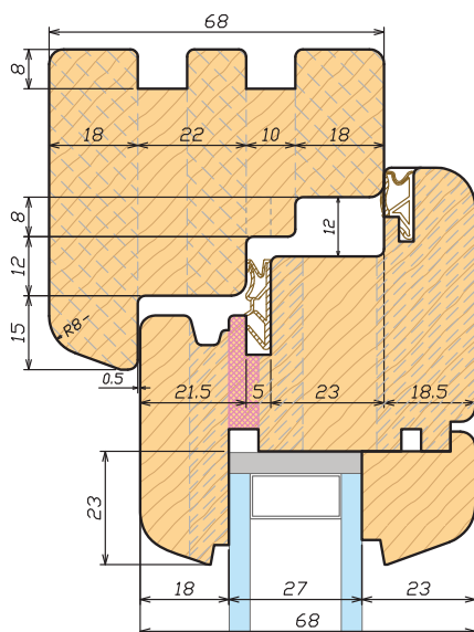
Sezione verticale 68 Vertical section 68
