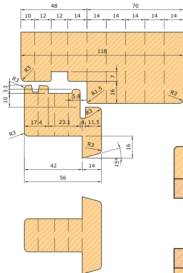
Sezione verticale Vertical section
