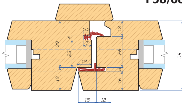
Sezione orizzontale - Chiusura centrale 58 Horizontal section - Central closure 58
