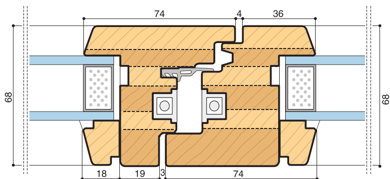
Sezione orizzontale - Chiusura centrale Horizontal section - Central closure
