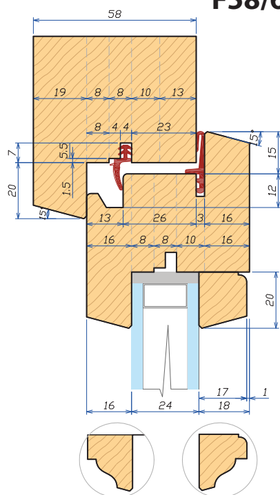
Sezione verticale 58 Vertical section 58
