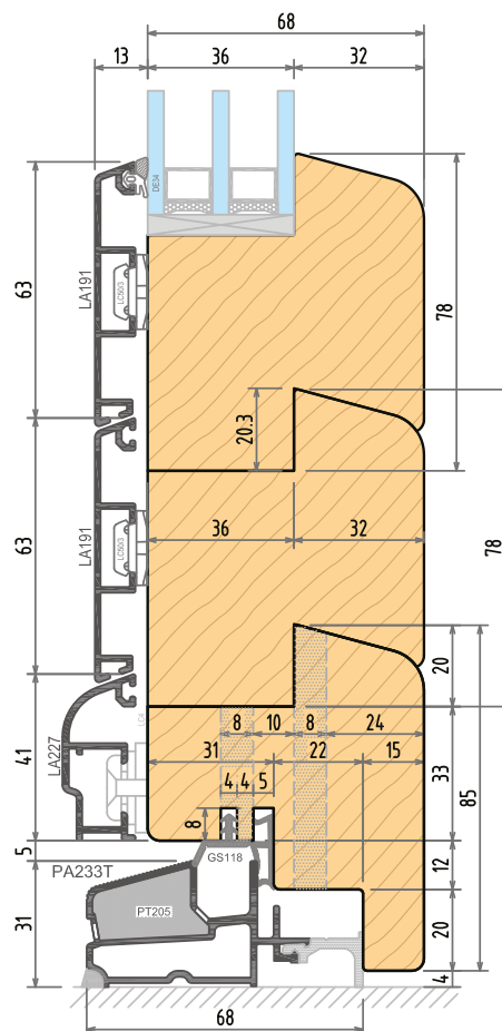
Sezione verticale - Portafinestra Vertical section - French door
