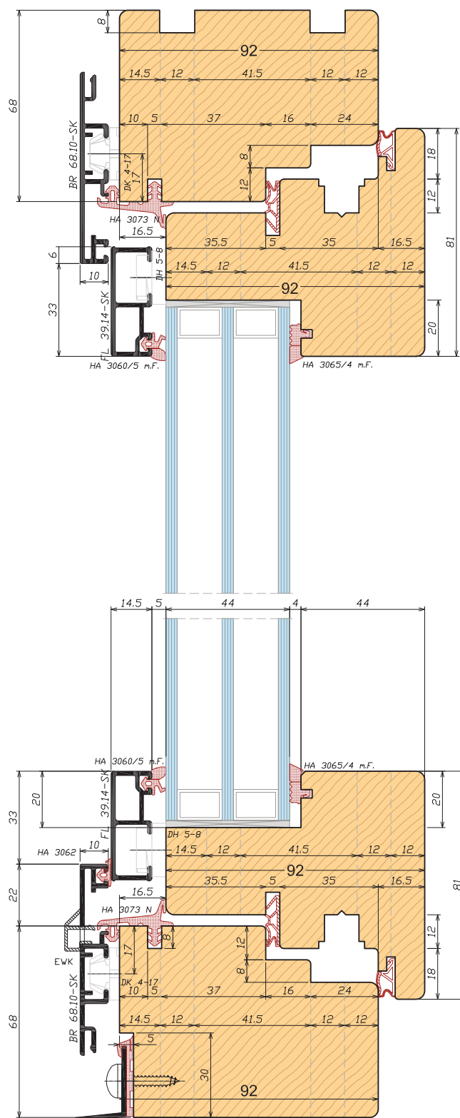
Sezione verticale Vertical section
