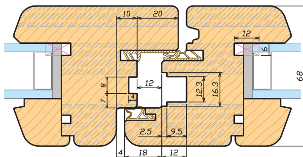
Sezione orizzontale - Chiusura centrale 68 Horizontal section - Central closure 68
