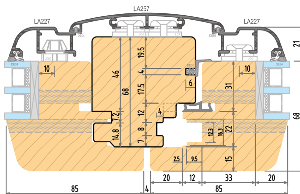
Montantino aggiuntivo Additional jamb
