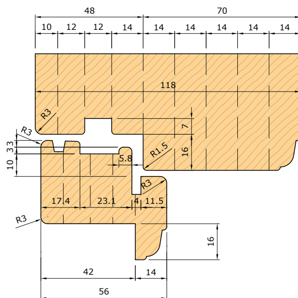
Sezione verticale Vertical section
