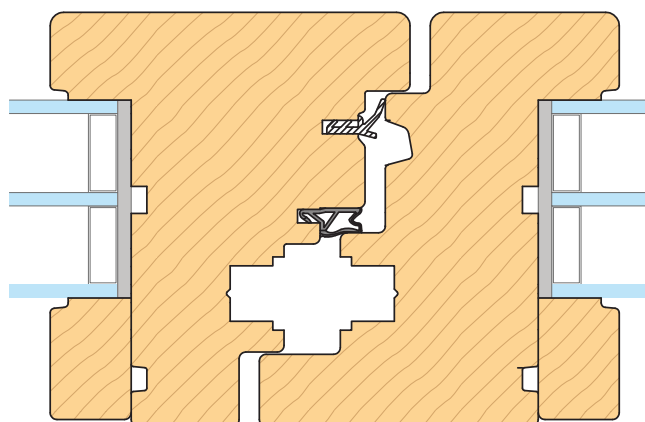
Sezione orizzontale - Chiusura centrale Horizontal section - Central closure
