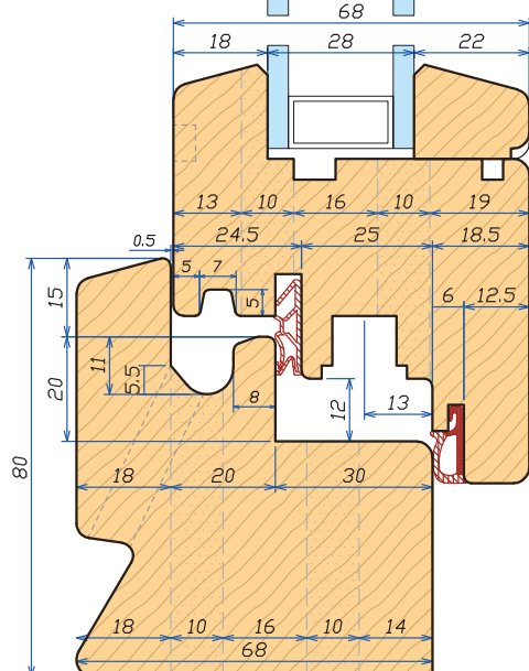
Sezione verticale Vertical section
