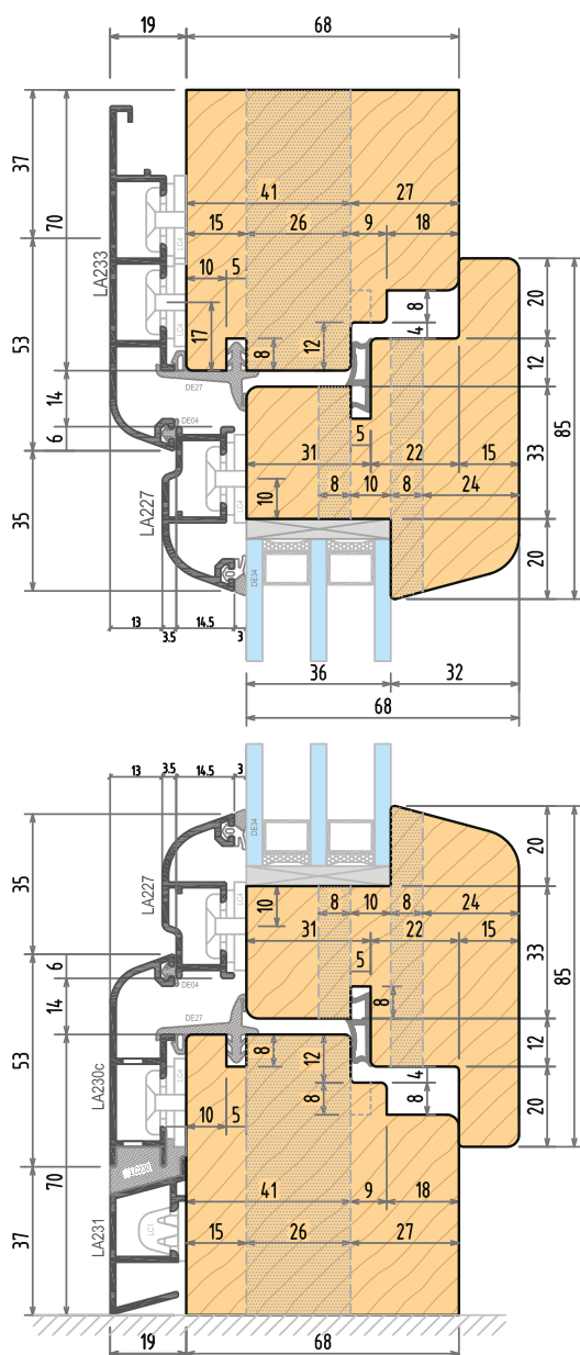
Sezione orizzontale chiusura centrale Horizontal section central closure
