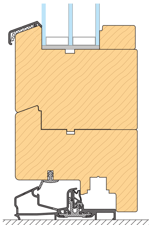
Sezione verticale - Portafinestra Vertical section - French door
