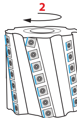
Spirale sinistra scarico del truciolo verso destra
