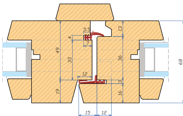
Sezione orizzontale - Chiusura centrale 68 Horizontal section - Central closure 68
