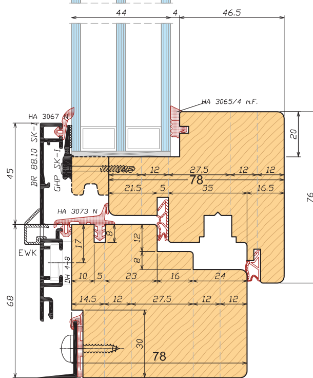
Sezione verticale Vertical section
