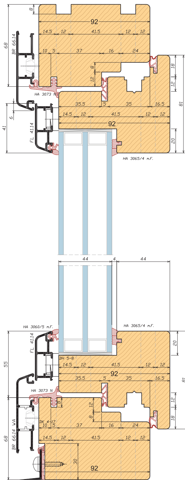
Sezione verticale Vertical section
