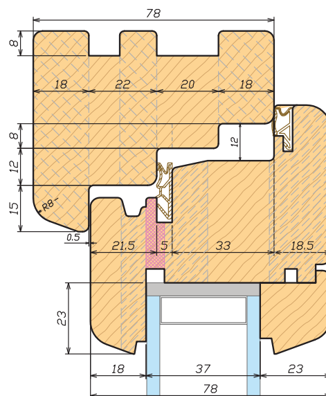
Sezione verticale 78 Vertical section 78
