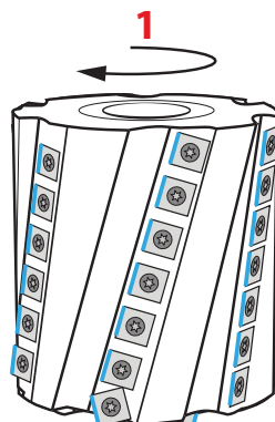
Spirale destra scarico del truciolo verso sinistra
