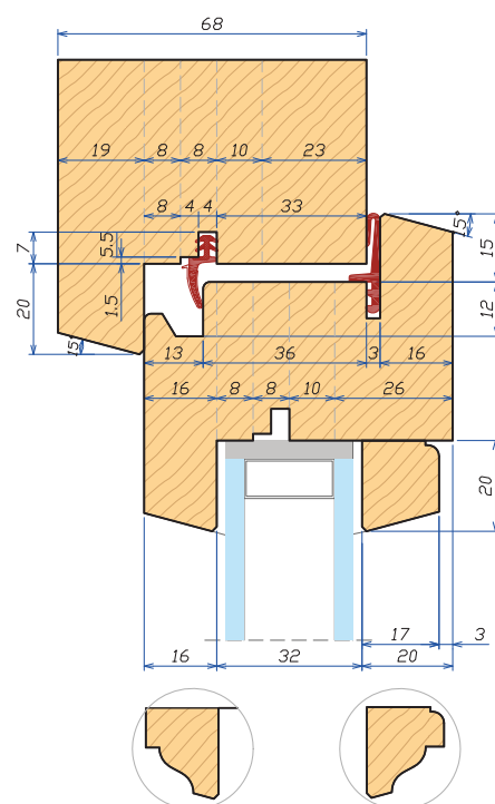
Sezione verticale 68 Vertical section 68
