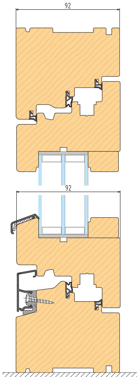
Sezione verticale Vertical section
