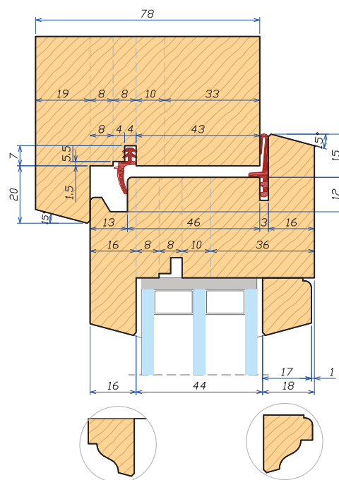
Sezione verticale 78 Vertical section 788
