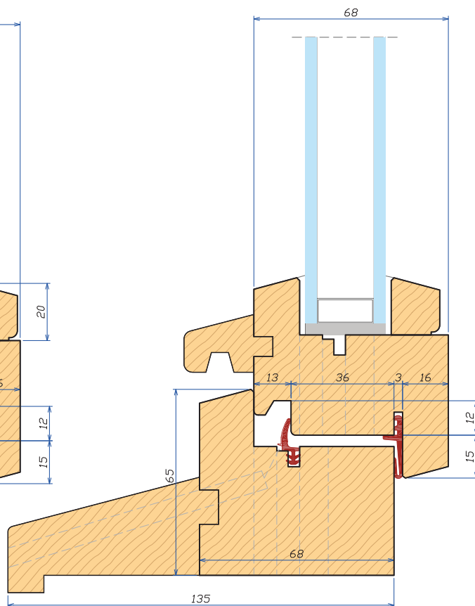
Sezione verticale 68 Vertical section 68
