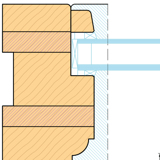
Sezione orizzontale Horizontal section
