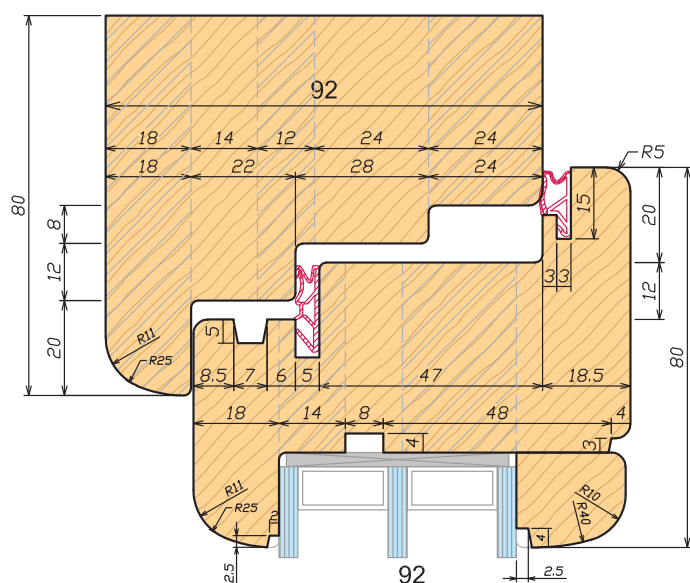
Sezione verticale Vertical section
