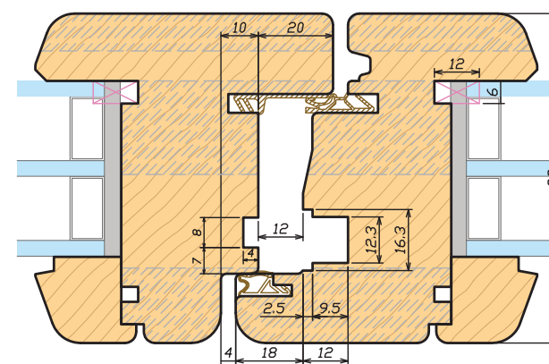
Sezione orizzontale - Chiusura centrale 88 Horizontal section - Central closure 88
