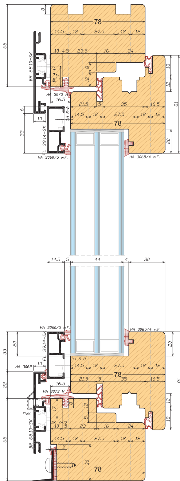
Sezione verticale Vertical section
