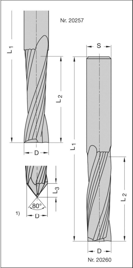
1) VHW-Bohrfräser für Durchgangsbohrungen siehe Seite 3.7
