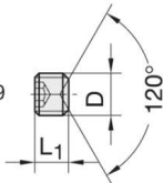
ISO 4029
