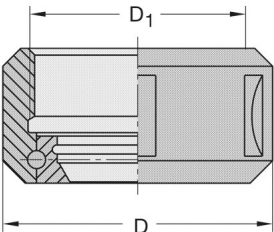
Spannmutter kugellagert 39042
